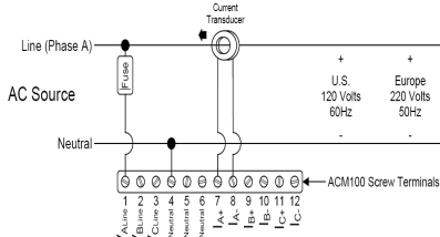
ACM100 i typisk enkelt fase applikation
