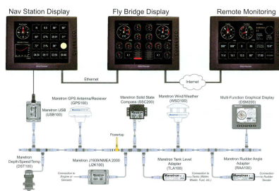
NMEA2000 netværk
