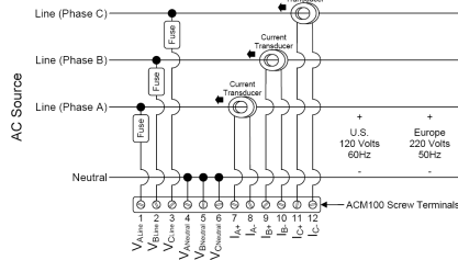
ACM100 i tre fase applikation
